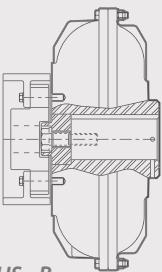
Type: HS..B
