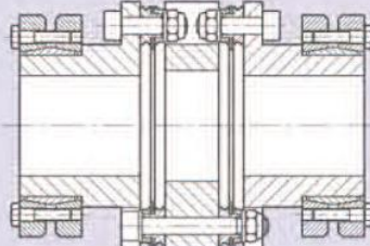
Type HH min
